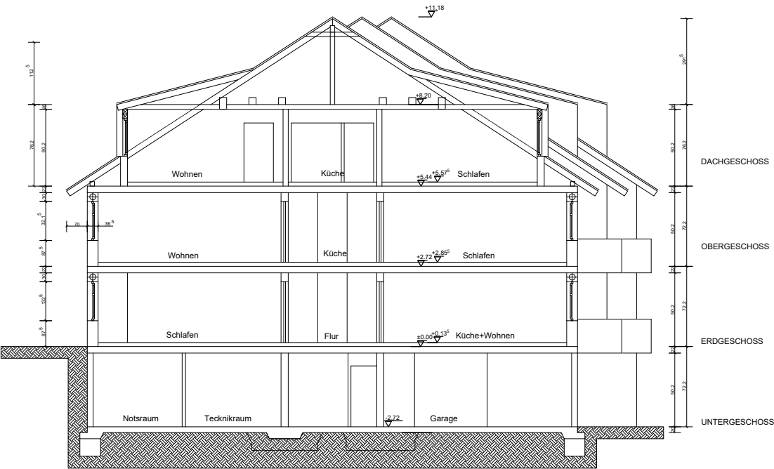
A-A SCHNITT
